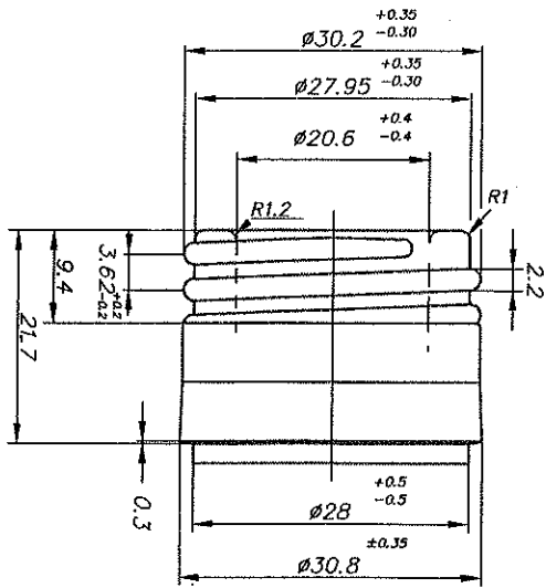
DETALJ GRLA NAVOJ R 2:1
